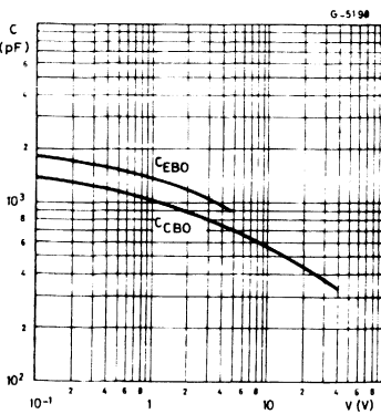
Capacitances (PNP types).
